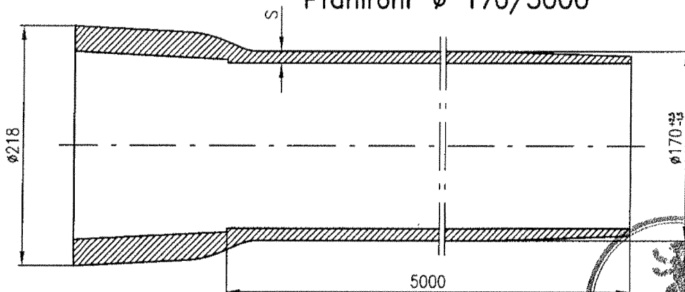
Pfahlrohr \varnothing 170/5000
