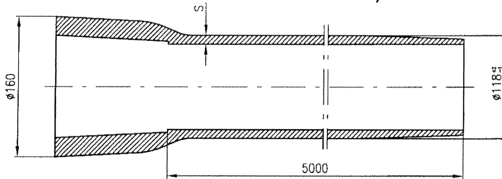
Pfahlrohr \varnothing 118/5000
